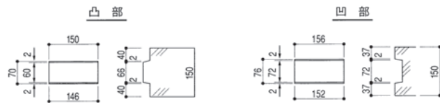
ジョイント詳細図
