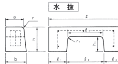
形状・寸法及び配筋図
